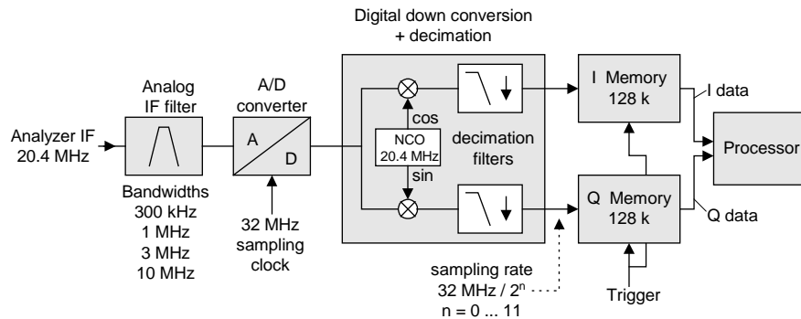
Blockschaltbild der Signalverarbeitung des Analyzers
