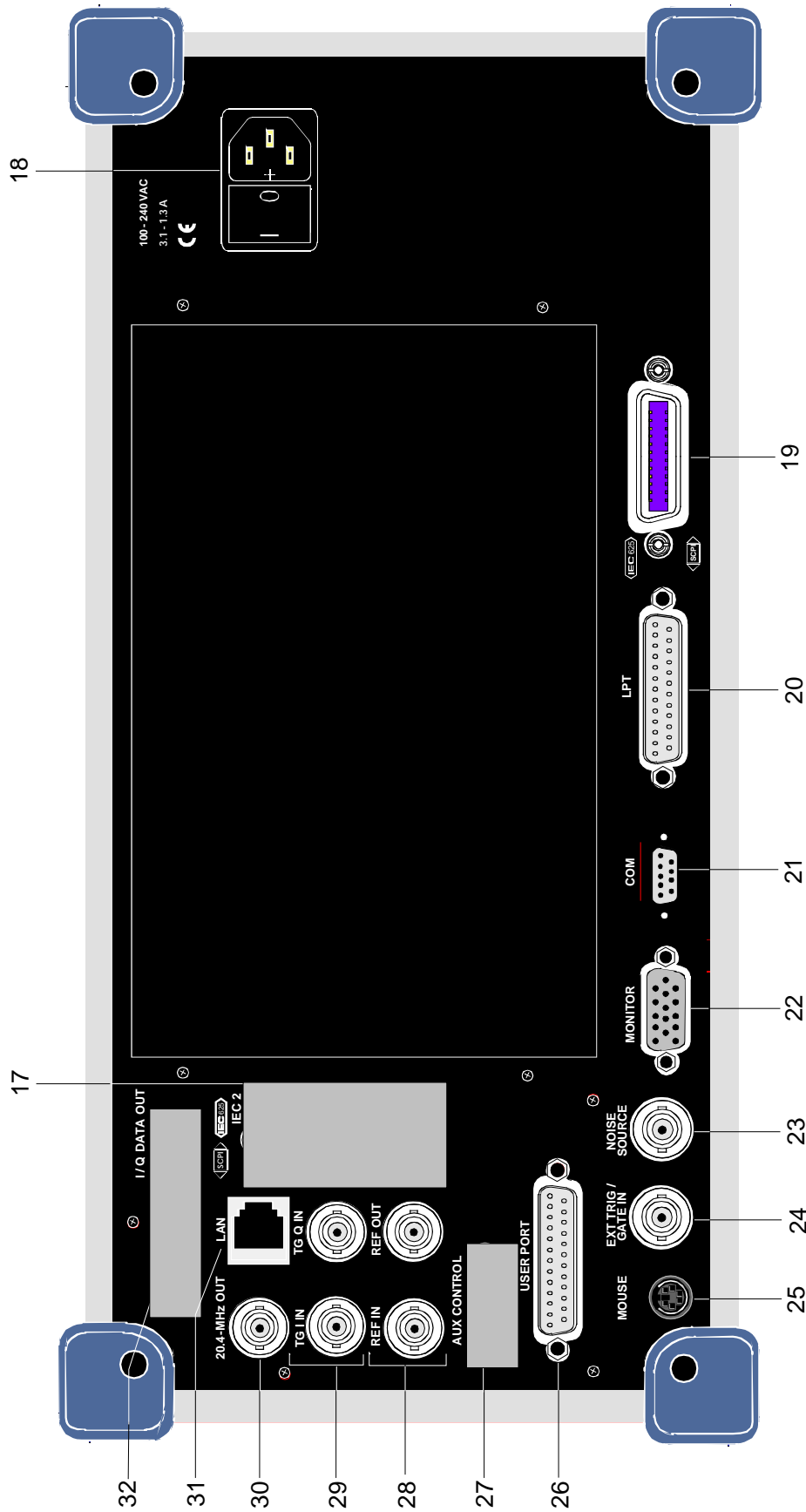
Bild 1-1 Rückansicht
