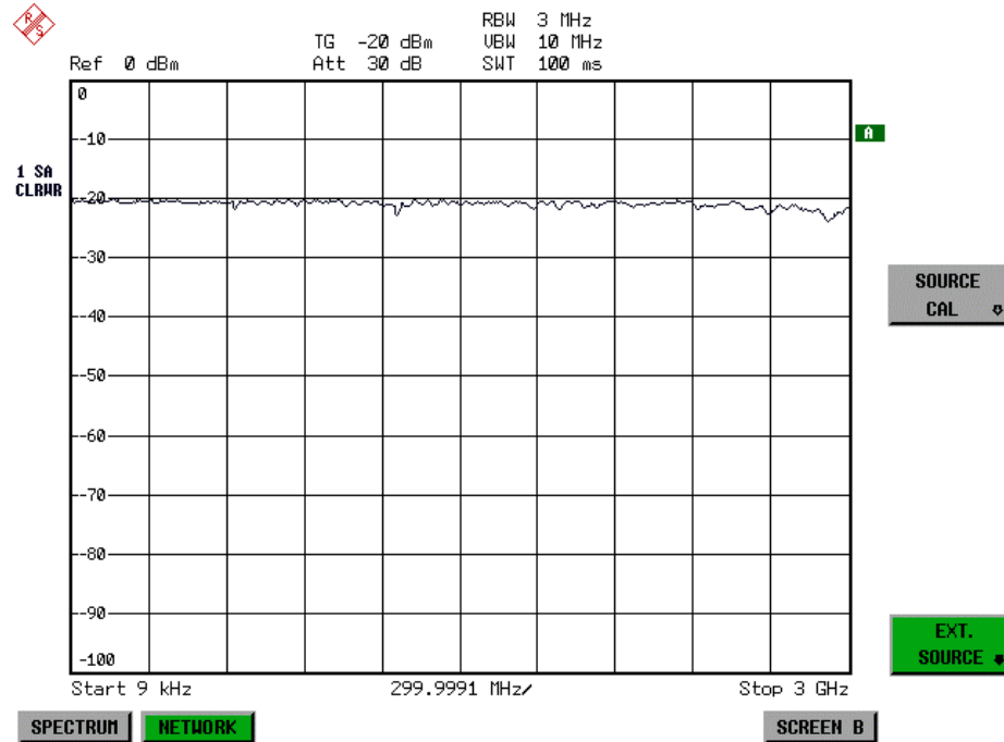
Bild 4-34 Meßkurve des Kalibriervorgangs einer Transmissionsmessung
