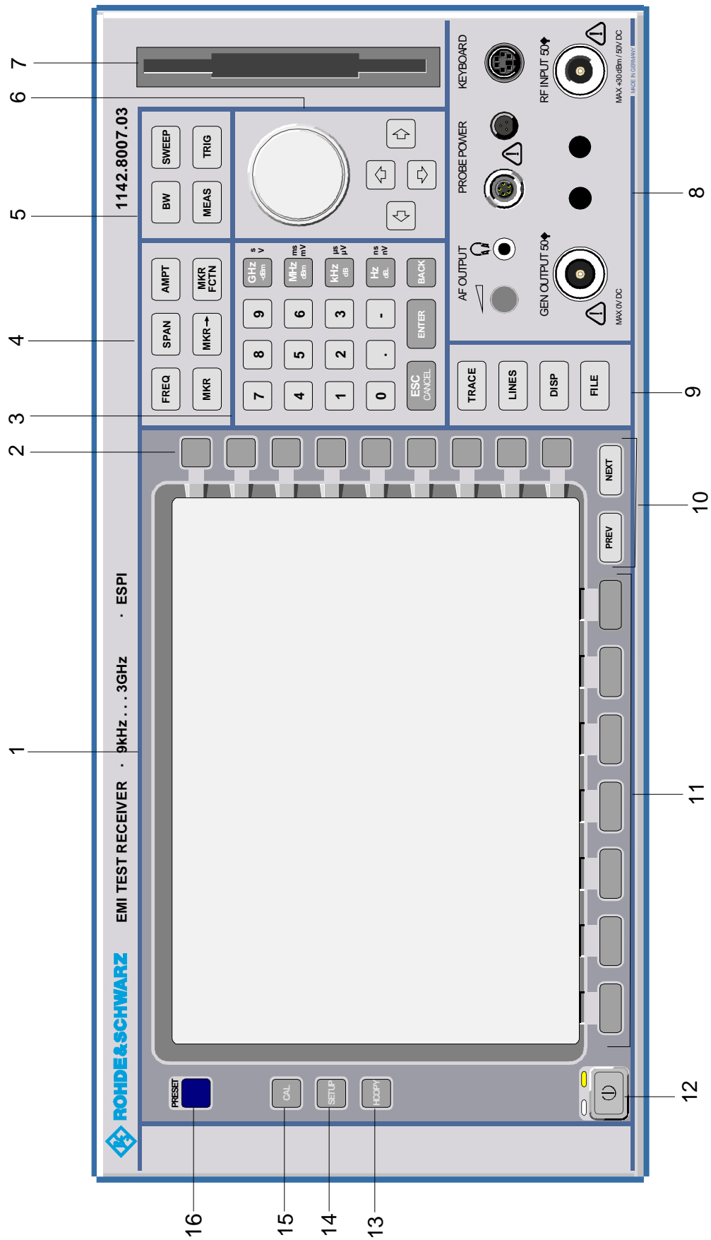
Bild 1-1 Frontansicht
